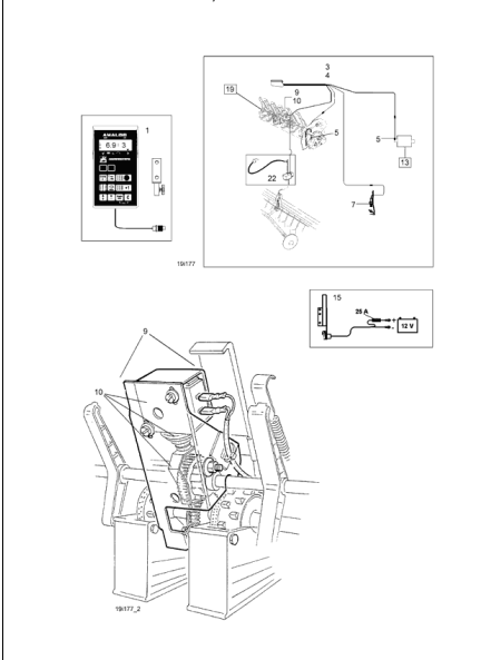
16 AMALOG, Kabelbaum f. AMALOG, Konsole m. Seite 34
